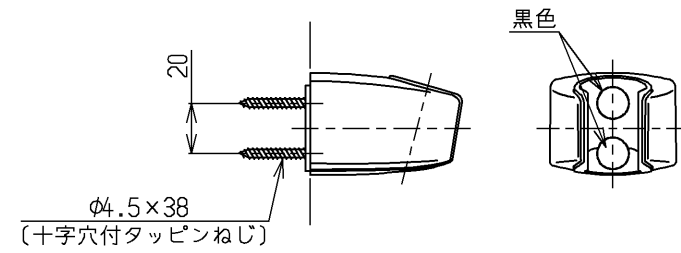
シャワーハンガー(2ヶ)
