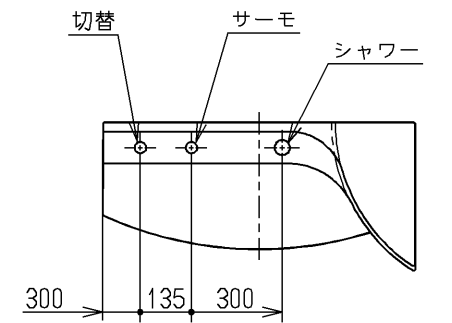
水栓取付け位置 (フリー)
