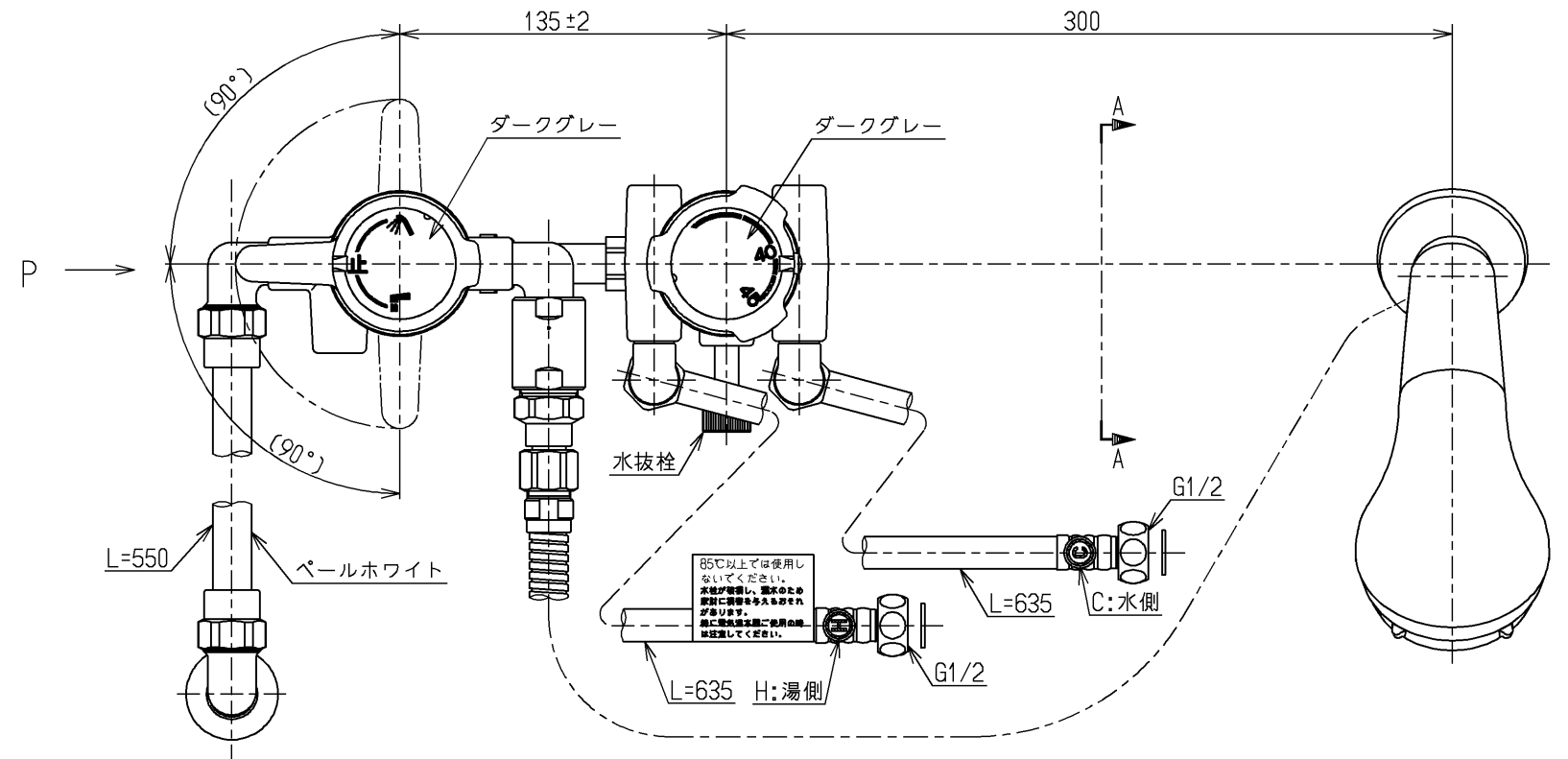
水栓取付け位置 (フリー)
